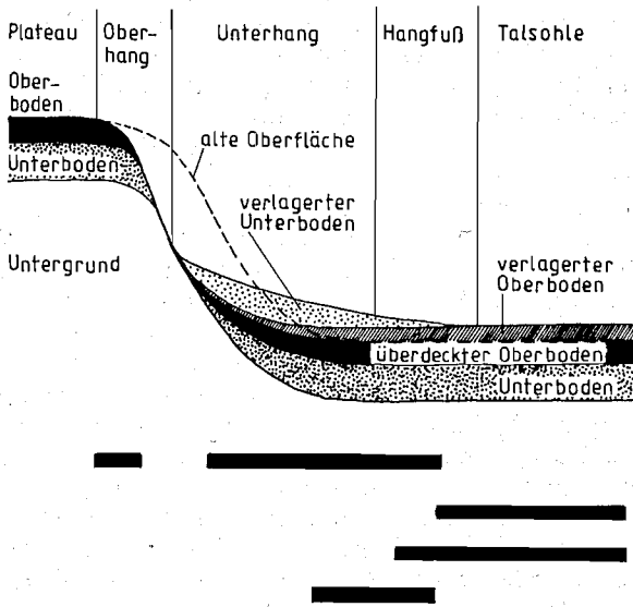
Abb. 2. Verteilung der in Abb. 1 erfaßten Regenwurmart an Hängen im Flußgebiet von Kokel und Mieresch. Schema der Hangcatena in Anlehnung an LIEBEROTH (1982)
