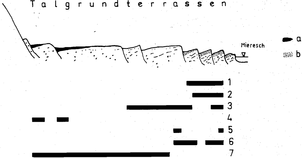
Abb. 1. Verteilung der stellenweise vorkommenden Regenwurmart des Mineralbodens in der Aue am Unterlauf des Mieresch. Schematisch vereinfacht
