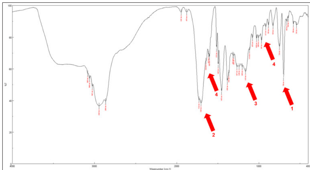
Abb. 15: Infrarotspektrum der Krantzit-Probe aus Amsdorf (IRS Nr. 933 Warszawa).
