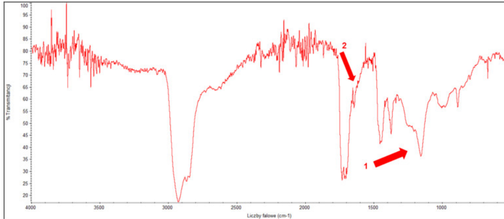
Abb. 16: Infrarotspektrum der Succinit-Probe aus Köplitz (IRS Nr. 5 PK Gdańsk).
