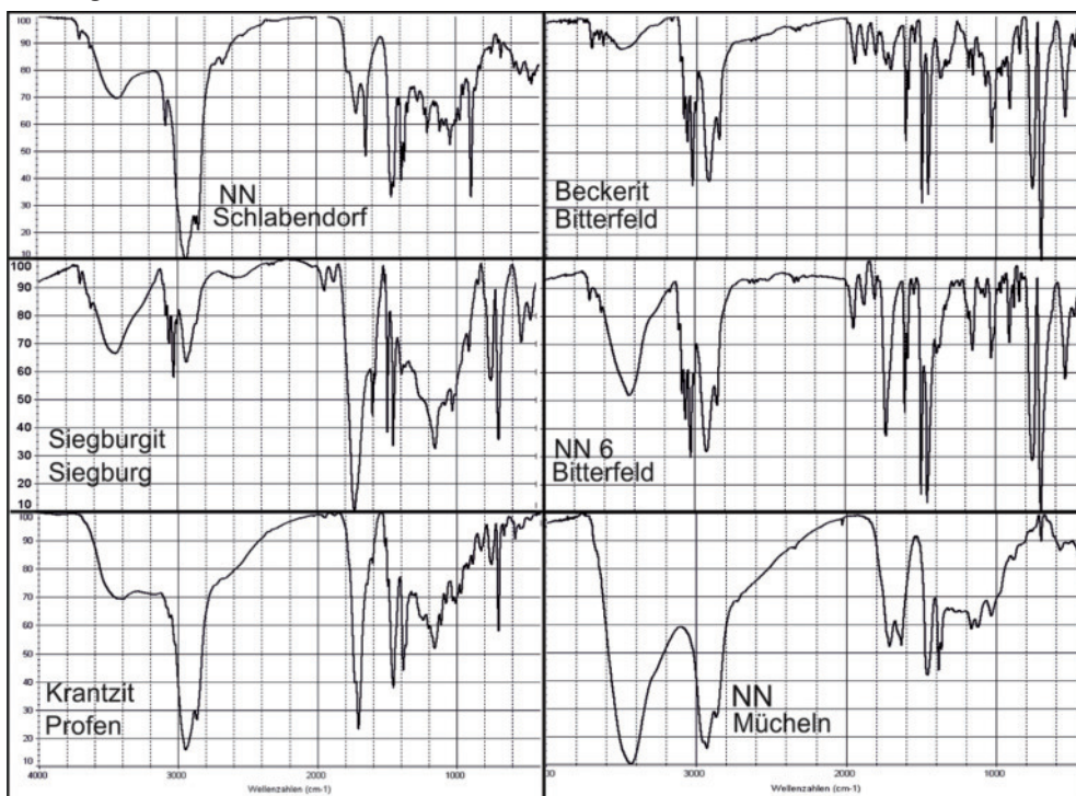
Abb. 3: Infrarotspektren (IRS) des miozänen Sandbernstens von Schlabendorf-Süd, des Sieburgit sowie mittelozäner Bernsteine im Vergleich mit einigen Bernsteinarten aus Bitterfeld.
