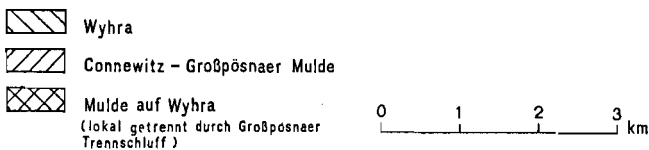
Abb.1 Verbreitung der frühelsterkaltzeitlichen Flußschotter im Raum Espenhain - Stormthal
