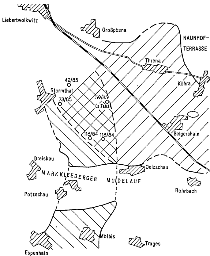
Abb.1 Verbreitung der frühelsterkaltzeitlichen Flußschotter im Raum Espenhain - Stormthal
