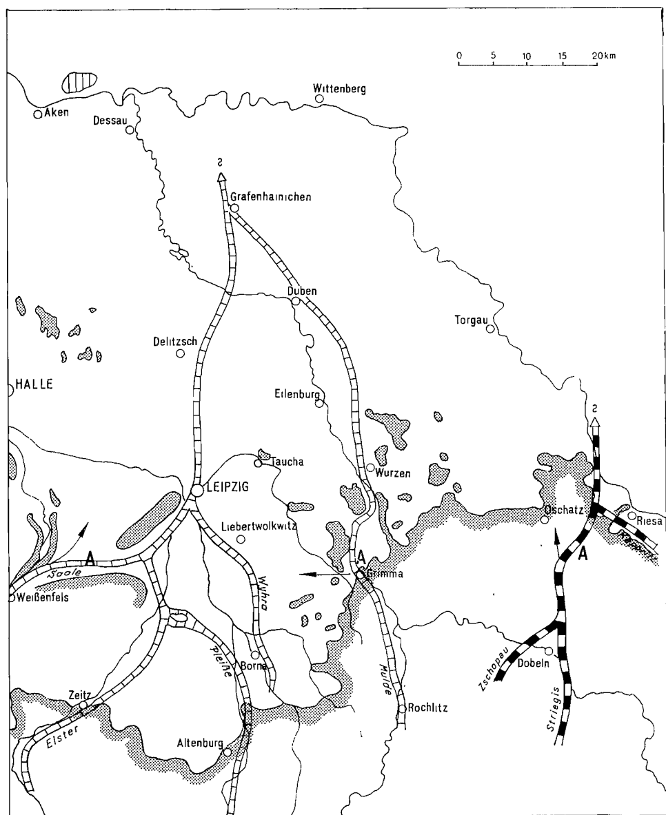
Abb 5: Darstellung des helmekaltzeitlichen Flußsystems im Bereich der Leipziger Tieflandsbucht
