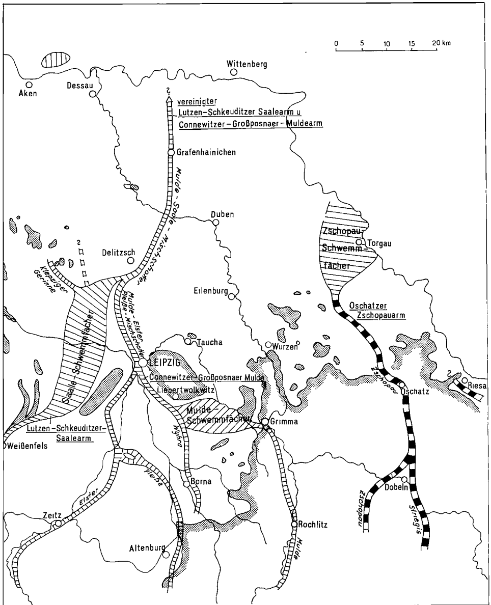
Abb. 6: Darstellung des frühelsterzeitlichen (im neueren Sinne) Flußsystems im Bereich der Leipziger Tieflandsbucht.
